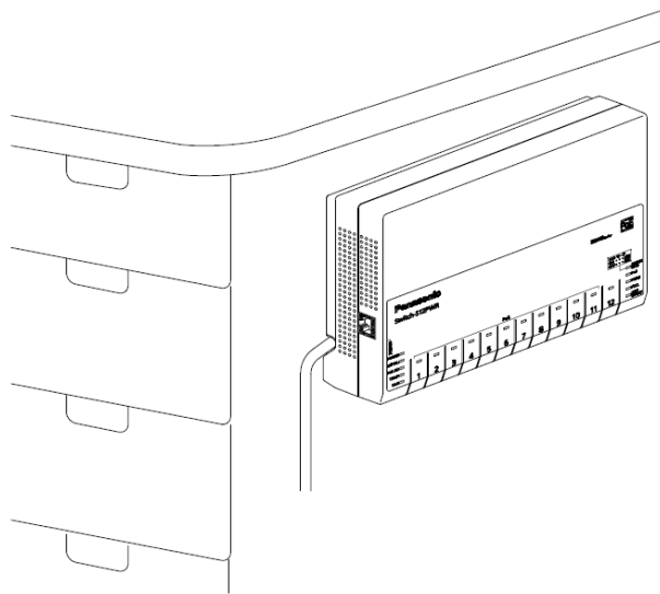
図2-1 スチール製製品への設置
