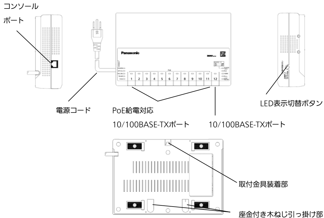
図1-4-1 Switch-S12PWR 外観図
