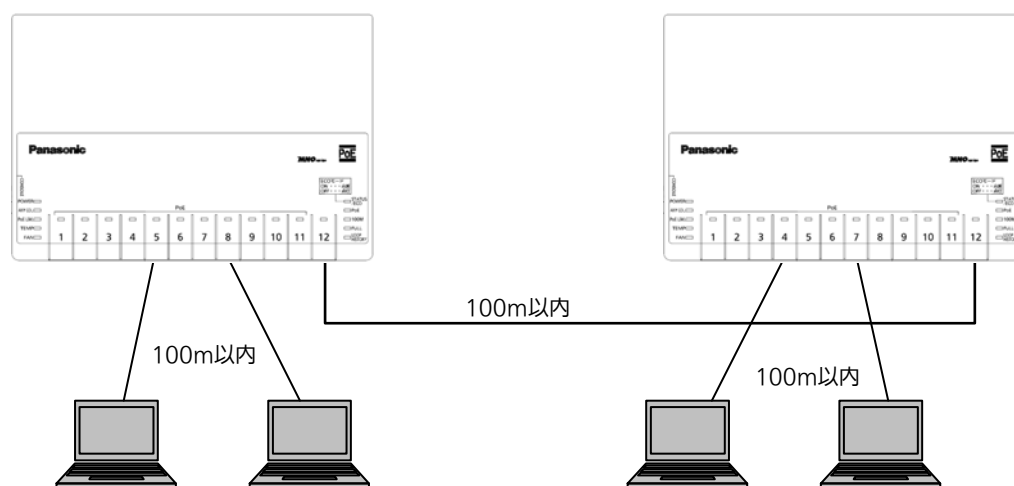
図3-1 接続構成例
