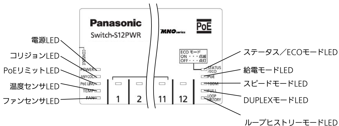
図1-4-2 前面パネル拡大図
