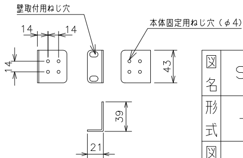
壁取付用金具 (同梱)
