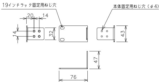
19インチラック固定用金具 (同梱)
